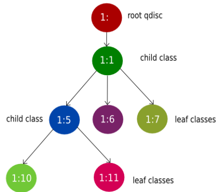
Figura 2: Ejemplo de árbol de clases en tc
