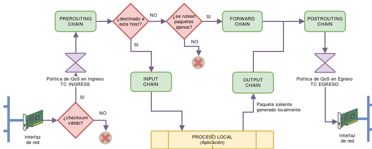
Figura 2: Esquema de funcionamiento de las interfaces de red de un equipo linux
